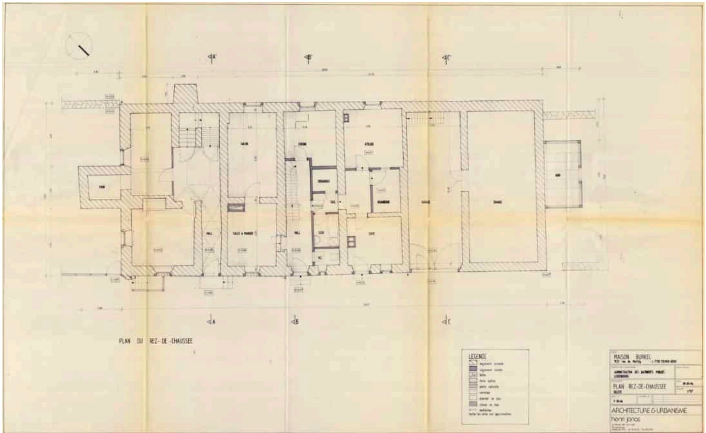
▲ Grundrissplan des Erdgeschosses des ehemaligen Bauernhofs 'A Burkels', 1994 Architecture & Urbanisme, Maison Burkels. Plan rez-de-chaussée, [Plan], erstellt von Henri Jonas, Administration des bâtiments publics (Luxemburg), Ettelbruck, 09.09.1994.
